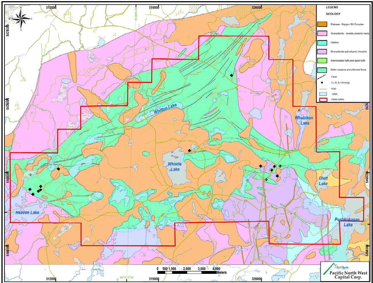
Abb. 2- Geologiekarte des Heaven Lake Projekts
