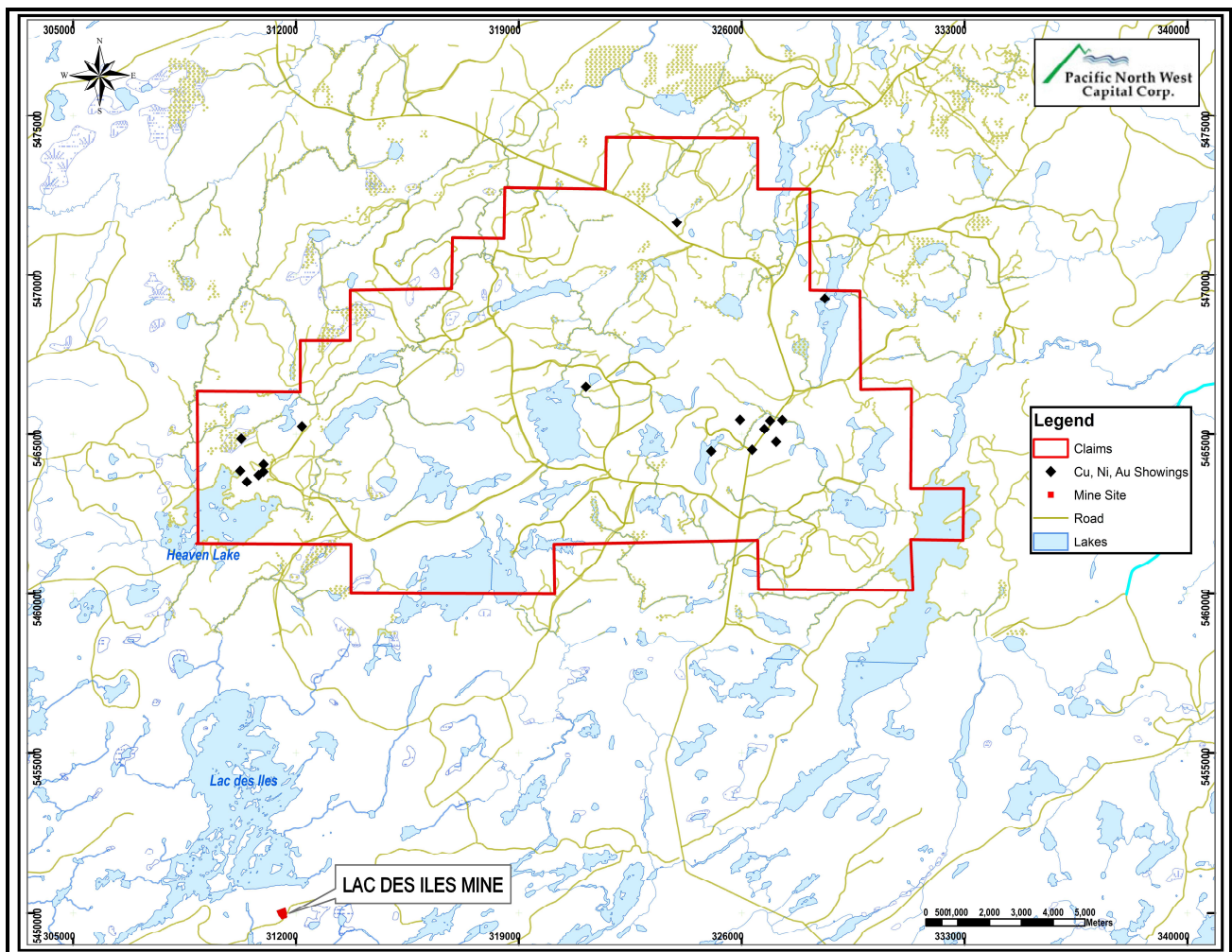
Abb.1 Lagenkarte des Heaven Lake Projekts
